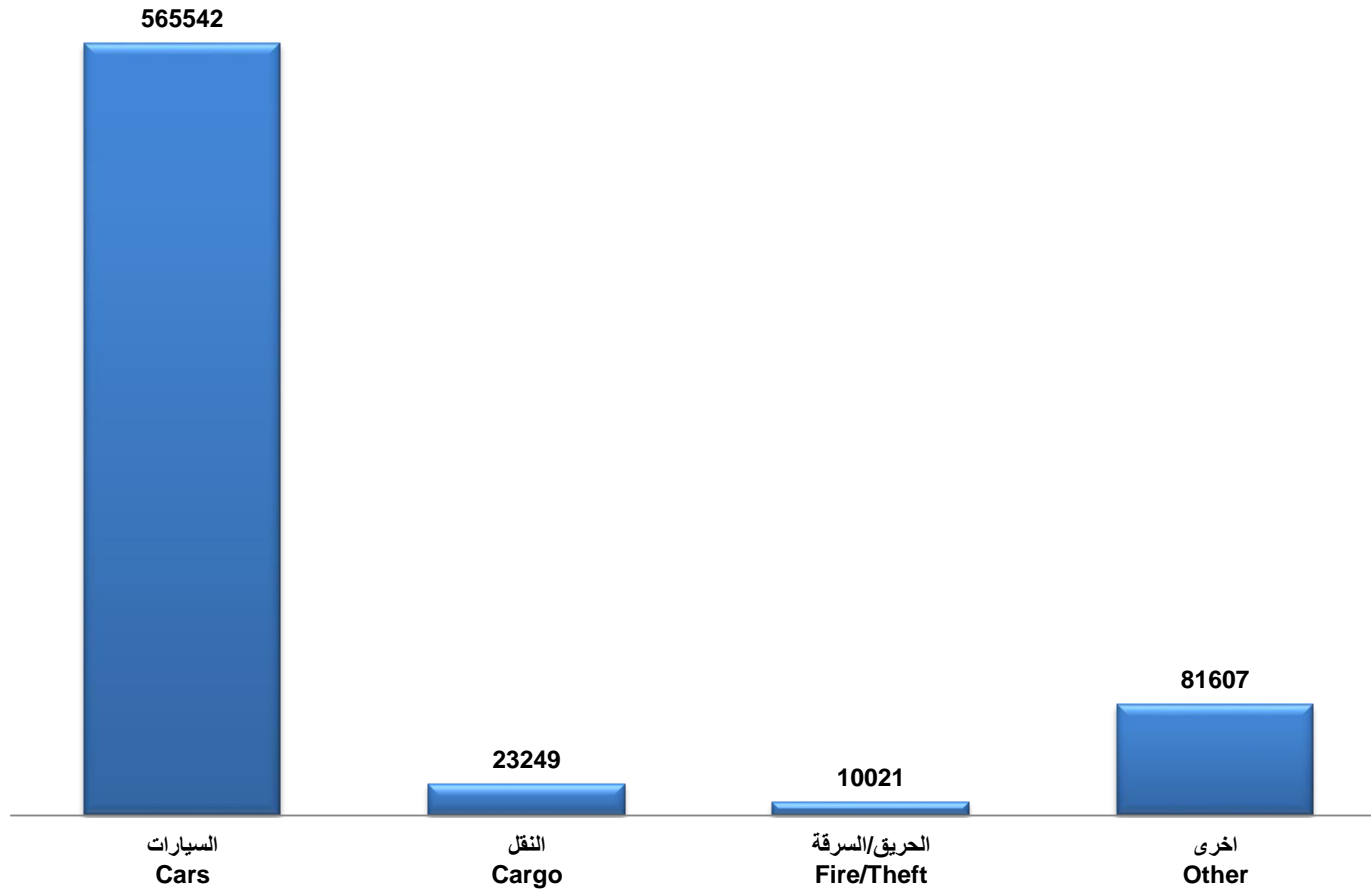
شكل (30) Graph
